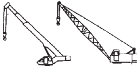
Estructura giratoria y pluma telescópica
